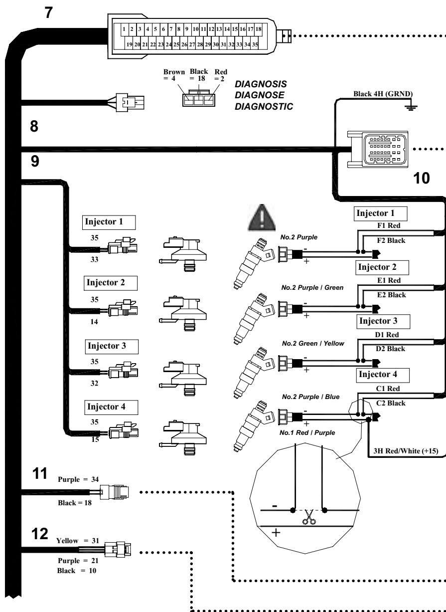
Cylinder arrangement / Cilindernummering Numérotage de cylindre Position of interruption / Plaats van onderbreking / Position du déconnection
