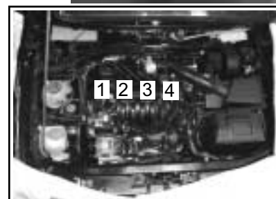
Cylinder arrangement / Cilindernummering Numérotage de cylindre Position of interruption / Plaats van onderbreking / Position du déconnection
