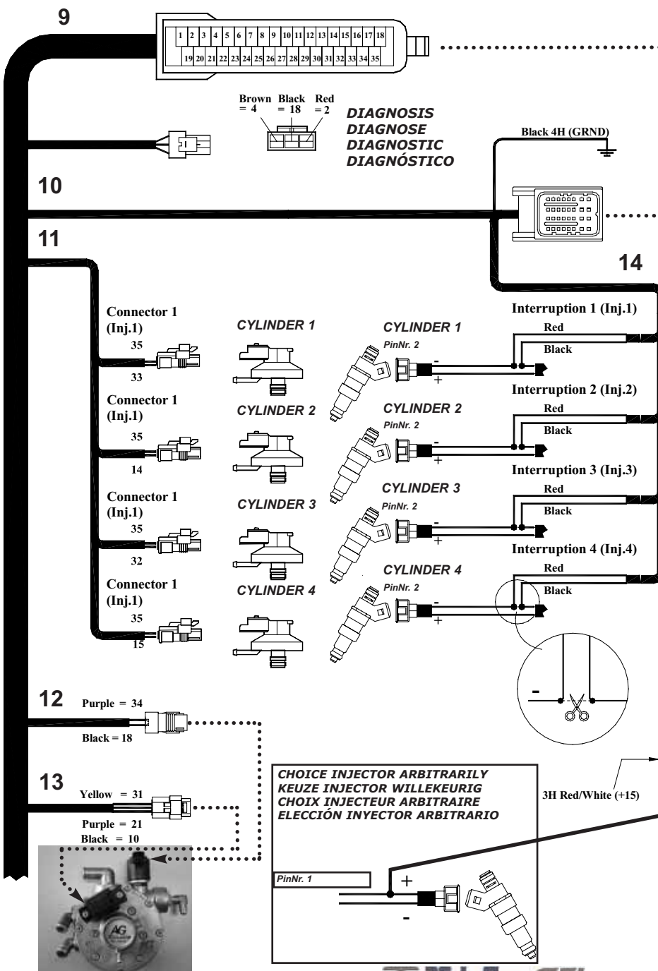
14 Cylinderarrangement / Cilindernummering Numérotage cylindre/Numeración cilindros
